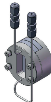
GS2056X 温度可変セル用シールフローセル
